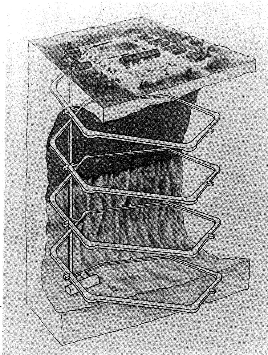
Figur 2.3 Översiktsbild av planerat berglaboratorium
