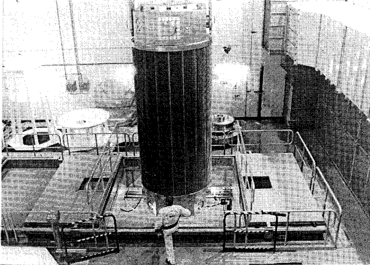
Hantering av transportbe- hållare i mottagningsdelen
