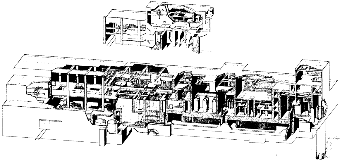
Figur 2.6 Behandlingsstation för använt bränsle
